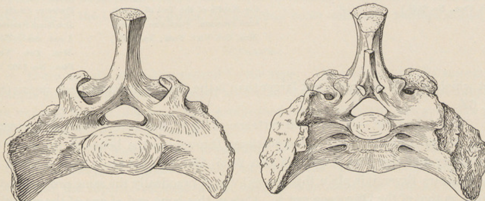
FIG. 61. Anterior and Posterior Views of Sacrum of D. hollandi Peterson. \frac{3}{4} nat. size. (Carn. Mus. Cat. Vert. Foss., No. 2126.)
