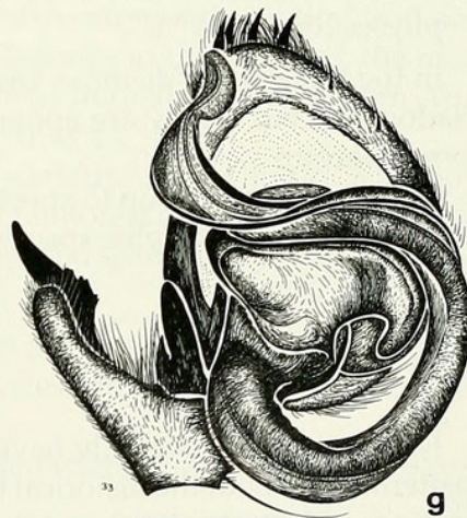
Fig. 3. Male palps of species of Storena from the formosa -group. a. S. recta . b. S. rotunda . c. S. aspinosa . d. S. fungina . e. S. martini . f. S. sinuosa . g. S. formosa . c: cymbium; dta: dorsal tibial apophysis; e: embolus; fl: flange; mvta: double membranous ventral tegular apophysis; vta: ventral tegular apophysis.
