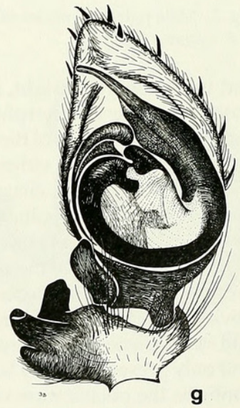
Fig. 1. Male palps of the most plesiomorphic species of Storena . a. S. procedens . b. S. digitulus . c. S. deserticola . d. S. ignava . e. S. raveni . f. S. mathematica . g. S. paucipunctata . dta: distal tegular apophysis; vta: ventral tegular apophysis.
