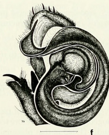
Fig. 3. Male palps of species of Storena from the formosa -group. a. S. recta . b. S. rotunda . c. S. aspinosa . d. S. fungina . e. S. martini . f. S. sinuosa . g. S. formosa . c: cymbium; dta: dorsal tibial apophysis; e: embolus; fl: flange; mvta: double membranous ventral tegular apophysis; vta: ventral tegular apophysis.
