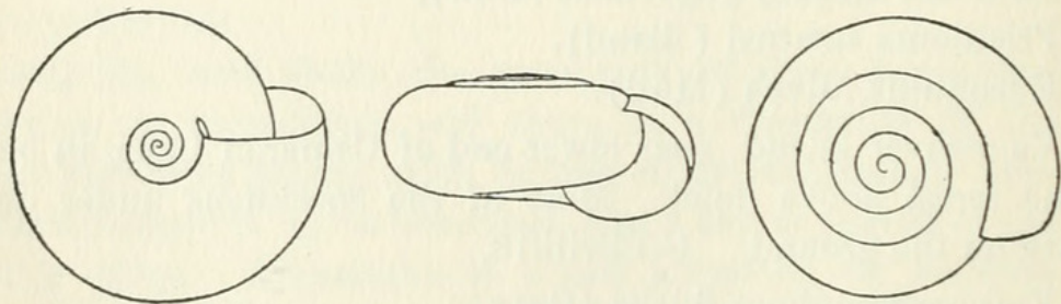
Fig. 1. Zonitoides cookei .
