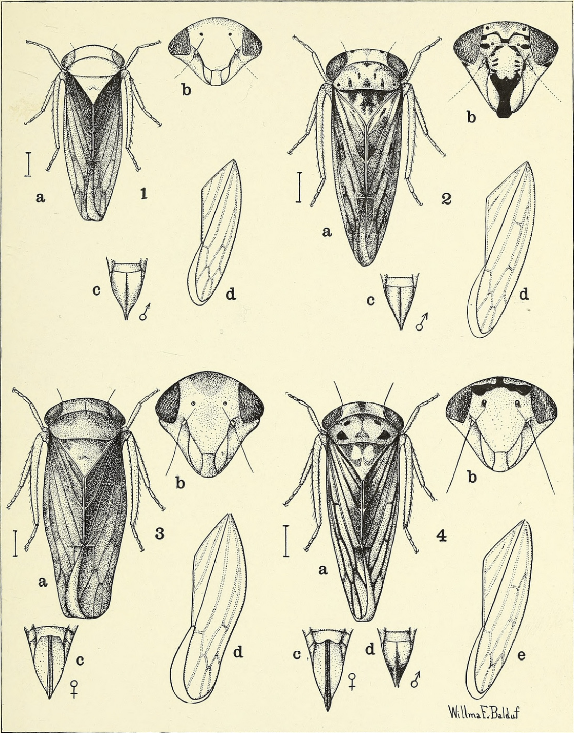
Idiocerus.
